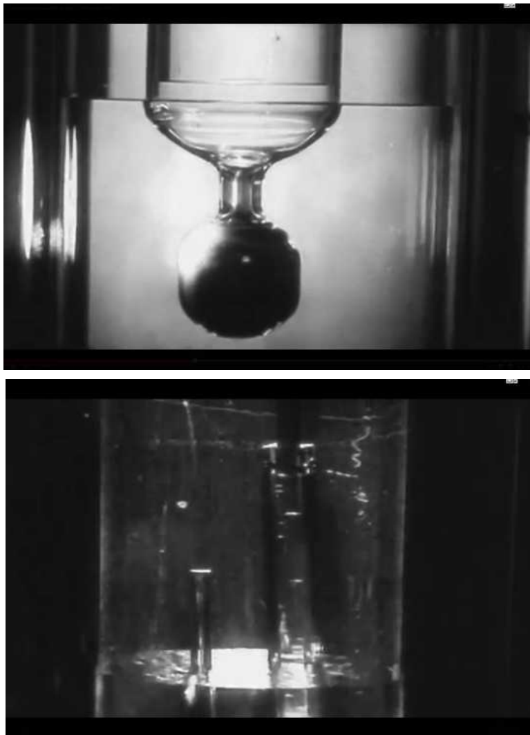
Рисунок 7 Фонтан-эффект (термомеханический эффект) в жидком гелии. Верхняя панель: подъём уровне гелия в трубке, закрытой снизу порошковой «пробкой» (тёмная расширенная часть трубки) при нагреве верхней части «пробки» сфокусированным излучением. Заполненная порошком часть трубки соединяется с жидким гелием в дьюаре через отверстие снизу. Повышение уровня жидкости в трубке над уровнем жидкости в дьюаре возникает только при нагреве. Нижняя панель: фонтан гелия, бьющий из капилляра при включении нагревателя. Кадры из демонстрационного фильма [3].
