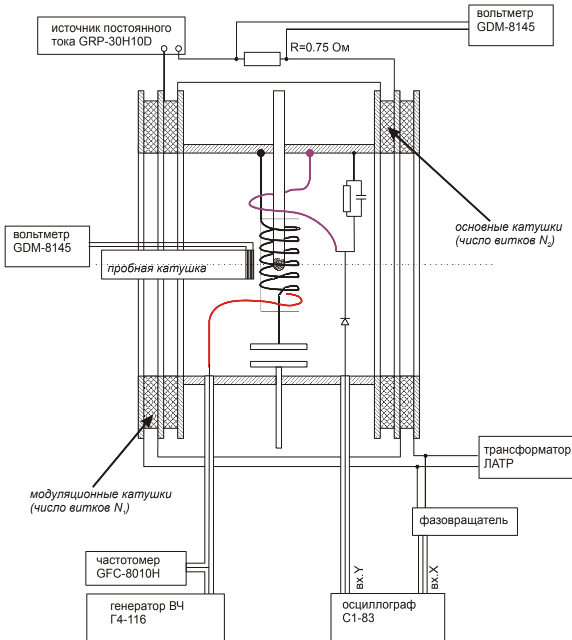
Рисунок 4: Схема установки.
