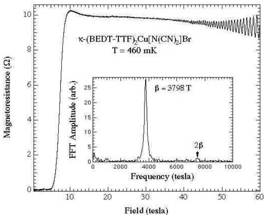
Рисунок 19: Осцилляции сопротивления в квазидвумерном проводнике \kappa -(BEDT-TTF) 2 Cu[N(CN) 2 ]Br в высоких магнитных полях до 60 Тл. На вставке — фурье-преобразование от наблюдаемых осцилляций. С сайта [13].
