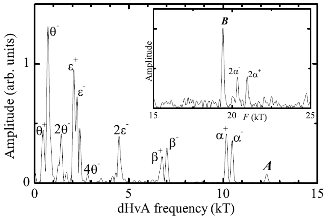
Рисунок 23: Осцилляции намагниченности в тяжелофермионном соединении CeCoGe_3 . Сверху: экспериментальные данные. Снизу: фурье-преобразование экспериментальных данных, показывающее наличие нескольких типов носителей заряда. T=60 мК, поле приложено под углом 9^\circ от оси [100] к оси [110] . Из статьи [16].
