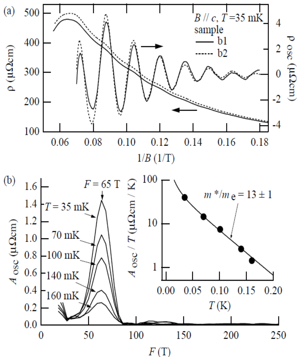
Рисунок 18: Пример наблюдения шубниковских осцилляций сопротивления в тяжелофермионном соединении \text{CeNiSn} . (a) Сопротивление как функция обратного поля при температуре 35 мК. Представлены данные измерений на двух образцах (сплошная и пунктирная линии). Также показана выделенная на фоне монотонного роста сопротивления в поле осциллирующая часть. (b) Преобразование Фурье от измеренной при разных температурах зависимости сопротивления. На вставке — зависимость амплитуды осцилляций от температуры. Из статьи [12].
