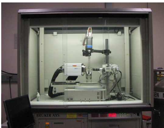
Рисунок 1 Слева: дифрактометр Bruker Smart Apex II (с сайта http://www.cif.iastate.edu/x-ray/apexii ). Справа: вид на образец в дифрактометре (фото автора). Справа налево по рис.: коллиматорная трубка, видеокамера, образец на гониометрической головке, полупроводниковый детектор.
