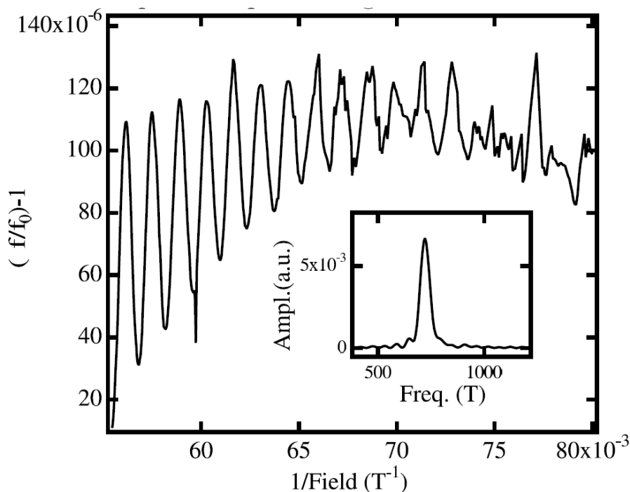
Рисунок 20: Осцилляции сопротивления в \kappa -(BEDT-TTF) 2 Cu(NCS) 2 , измеренные при давлении 1.67 кбар и температуре 90 мК в поле до 20 Тл. На вставке — фурье-преобразование осцилляций. Измерения проводились бесконтактным методом по изменению поверхностного высокочастотного импеданса. По вертикальной оси отложена частота высокочастотной колебательной системы. Из работы [17].
