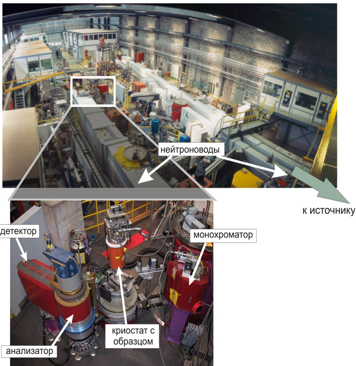
Рисунок 6: Экспериментальный зал источника нейтронов SINQ Института Поля Шерера (Виллиген, Швейцария). С сайта [4].
