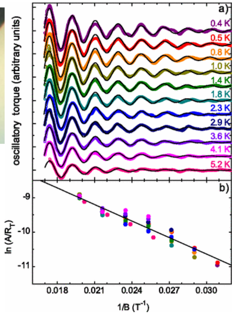
Рисунок 22: Слева: Образец сверхпроводящего купрата YBa_2Cu_3O_{6.5} на консоли магнетометра, размер образца 140 \times 140 \times 40 мкм 3 . Справа: осцилляции намагниченности в поле до 67 Тл и зависимость приведённой амплитуды осцилляций от поля. Чёрные кривые на левой панели — модельный расчёт в теории Лифшица-Косевича. С сайта [14] и из статьи [15].
