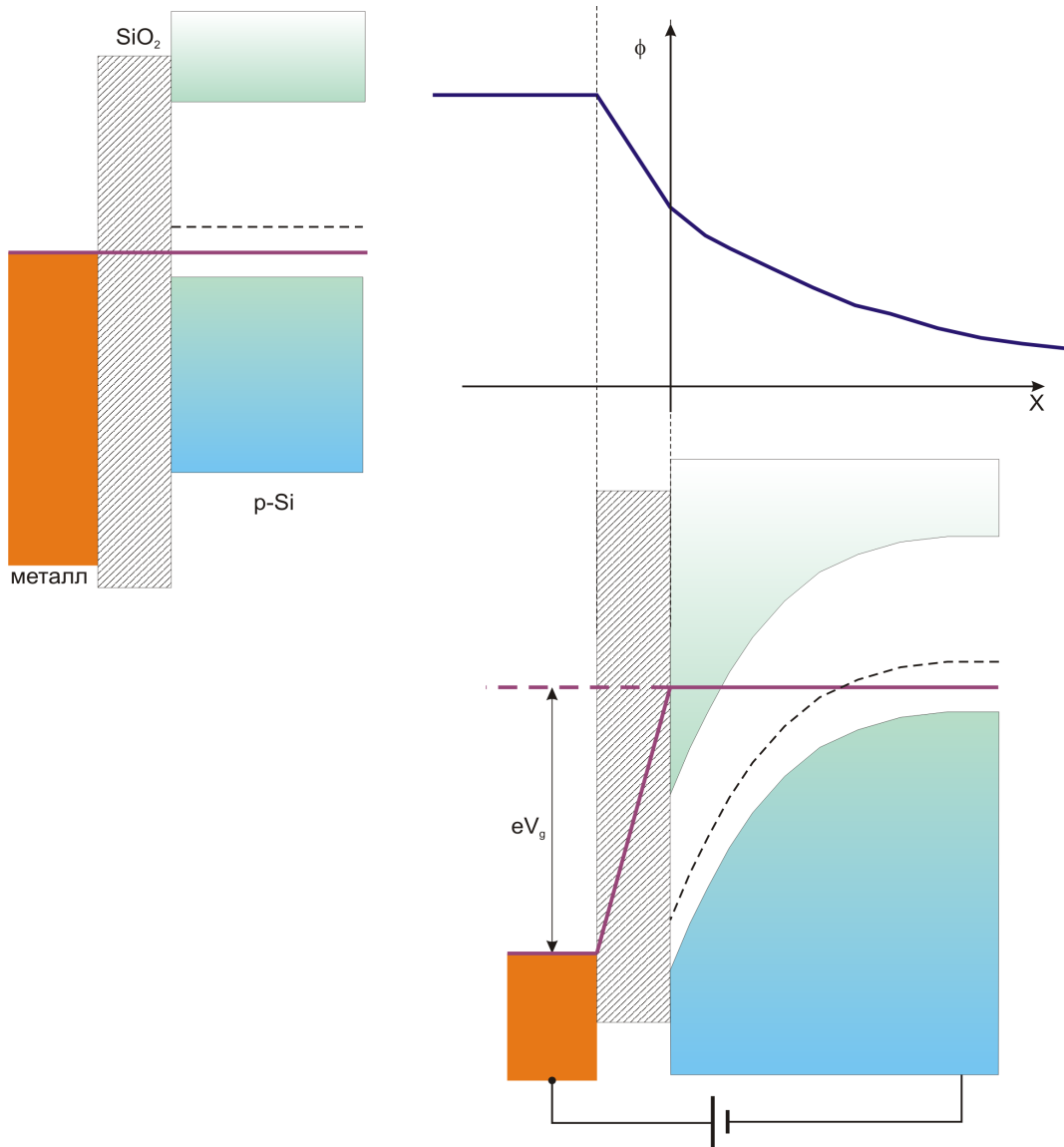
Рисунок 12: Энергетическая диаграмма полевого транзистора. Слева сверху: при равных потенциалах полупроводника и металла. Справа сверху: зависимость электрического потенциала от расстояния от границы при приложении к МОП-структуре внешнего напряжения (положительный потенциал металла). Справа внизу: представление энергетической диаграммы для полной энергии.
