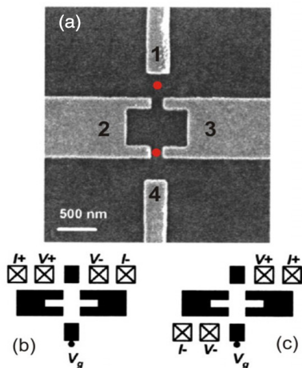
Рисунок 10 Сверху: Микрофотография (сканирующая электронная микроскопия) затворов на гетероструктуре из прибора, использовавшегося в опытах по квантованию одномерной проводимости. Снизу: две конфигурации эксперимента с таким прибором. Конфигурация с током через одномерный контакт (b) и через квантовую точку (c). Из обзорной статьи [18].
