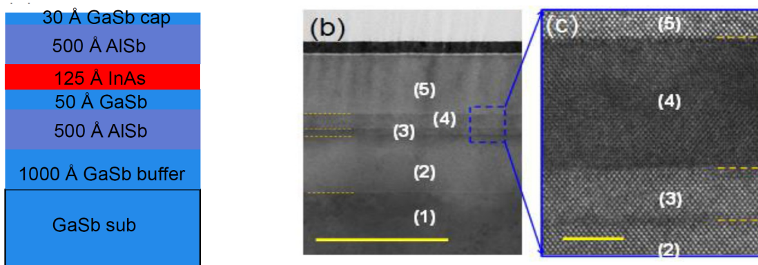
Рисунок 11 Слева: схема чередования слоёв в сложной гетероструктуре. Красным цветом выделен слой InAs, в котором формируется потенциальная яма для электронов. В центре и справа: изображения (туннельная электронная микроскопия) среза реальной гетероструктуры. Горизонтальная жёлтая линия задаёт масштаб, она равна 100 нм для центрального рисунка и 5 нм для правого. Жёлтый пунктир показывает границы слоёв. Нумерация слоёв: (1) буферный слой GaSb, (2) AlSb, (3) GaSb (потенциальная яма для дырок), (4) InAs (потенциальная яма для электронов), (5) AlSb. Из работы [19].
