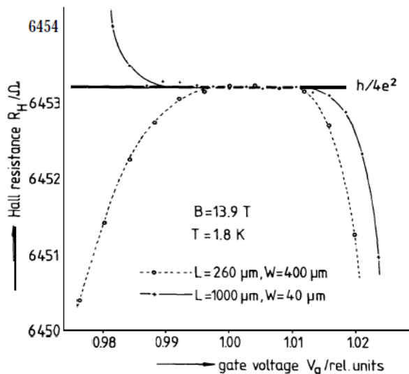
Рисунок 31: Сравнение плато Холловского сопротивления для образцов разной формы ( L - длина, W - ширина). На графике изображена зависимость холловского сопротивления от напряжения на затворе МОП-структуры, контролирующего концентрацию электронов в двумерном газе. Из статьи [5].
