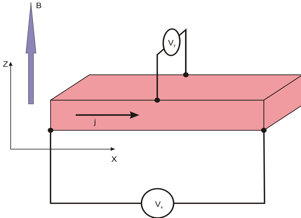
Рисунок 22: Схема опыта по измерению классического эффекта Холла.
