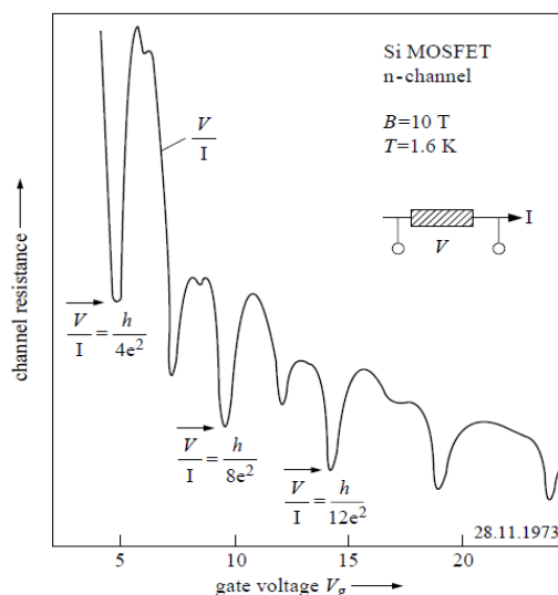
Рисунок 33: Зависимость двухконтактного сопротивления в цепи сток-исток МОП-транзистора от напряжения на затворе ( B=10T , T=2K ). Из статьи [6].
