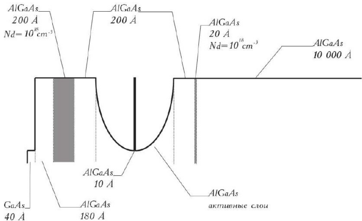
Рисунок 13: Пример гетероструктуры, в которой формируется параболическая яма с узким барьером. Заштрихованные слои показывают области с донорным допированием, являющиеся источниками электронов для активной части структуры. Из книги [3].
