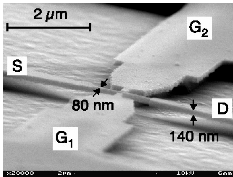
Рисунок 8 Полученное при помощи сканирующего электронного микроскопа изображение свободно подвешенного кремниевого «квантового провода». Обозначения: S и D — источник и сток, G1 и G2 — затворы. С сайта [17].
