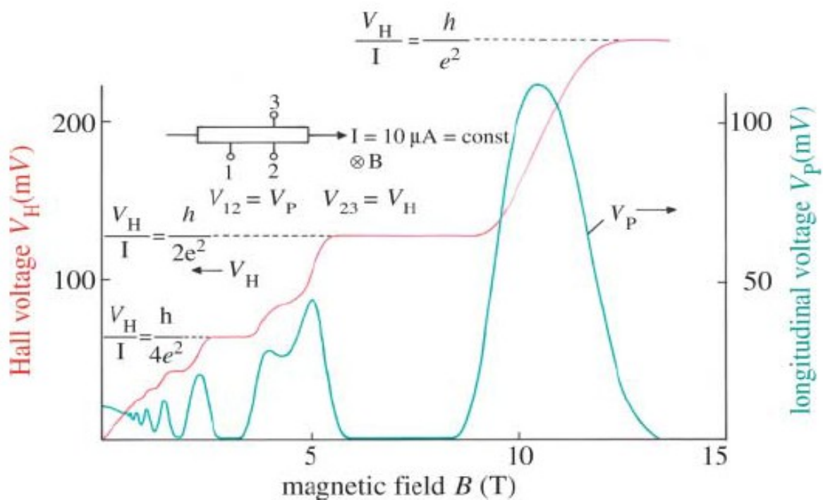
Рисунок 30: Зависимости от магнитного поля продольного и холловского напряжений на гетероструктуре GaAs-AlGaAs при токе 10 мкА. T=1.6 K . Из статьи [6].
