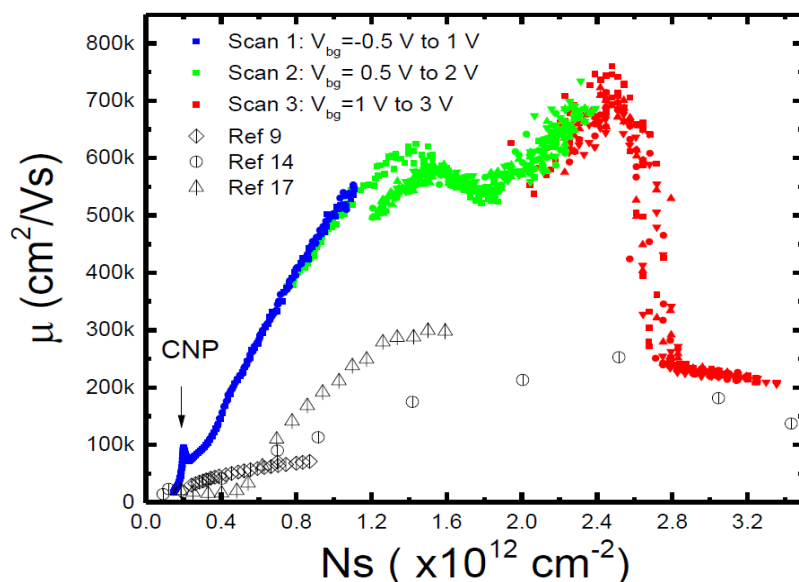
Рисунок 12 Зависимость подвижности электронов от концентрации носителей в гетероструктуре, показанной на рисунке 11. Из работы [19].
