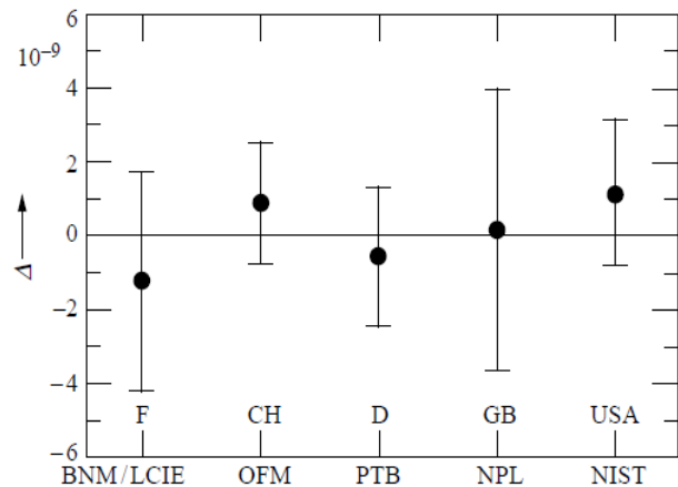
Рисунок 32: Воспроизводимость холловского сопротивления в различных лабораториях. Из статьи [6].
