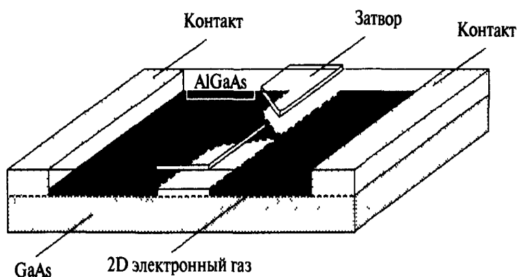
Рисунок 9: Схематическое изображение квантового микромостика. Черным цветом схематически отмечена область, в которой существует двумерный электронный газ. Из книги [1].
