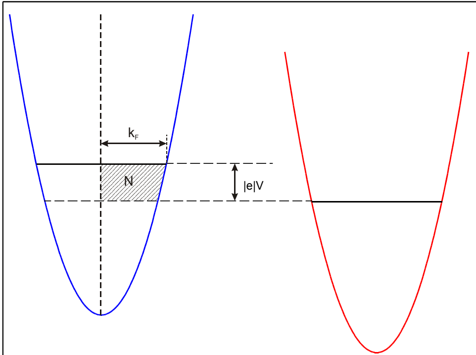
Рисунок 19: Зонная схема электронных состояний слева и справа от проводника. Штриховкой показаны состояния, участвующие в переносе заряда по проводнику.
