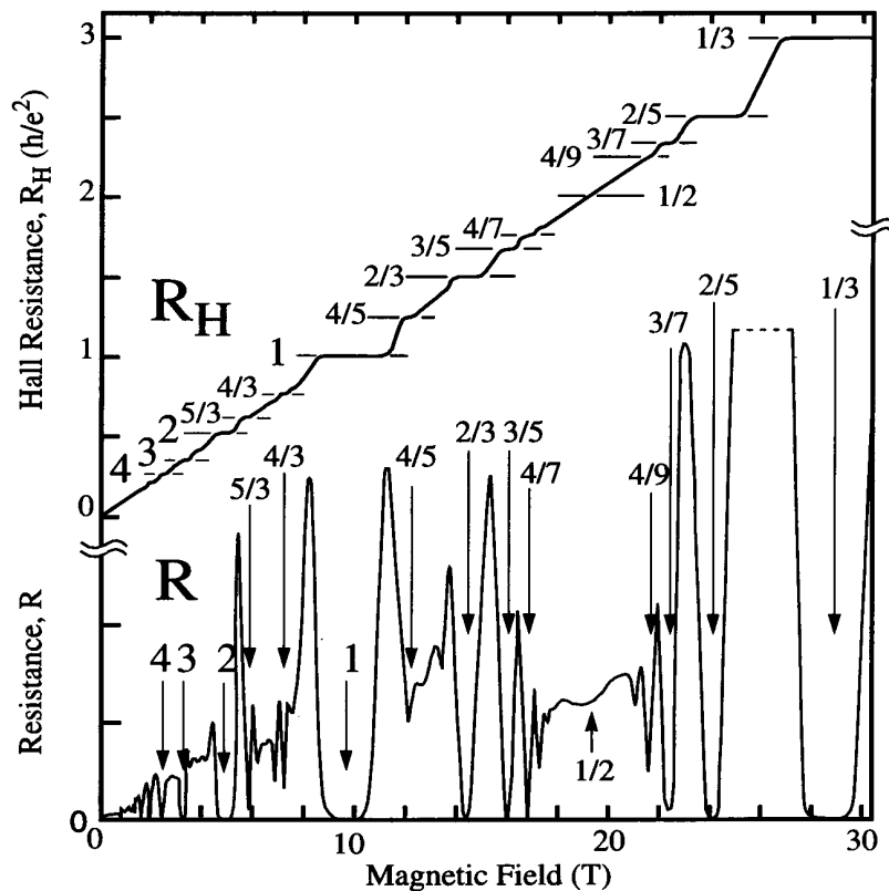
Рисунок 34: Наблюдение дробного квантового эффекта Холла в гетероструктуре GaAs-AlGaAs с высокой подвижностью носителей. Из статьи [23].
