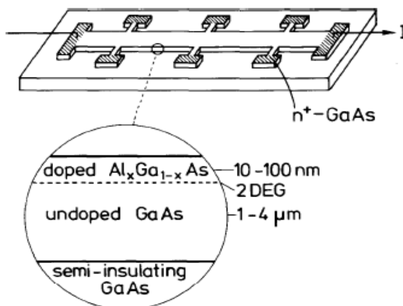
Рисунок 29: Форма и характерные размеры GaAs-AlGaAs гетероструктуры, используемой в опытах по квантовому эффекту Холла. Из статьи [5].
