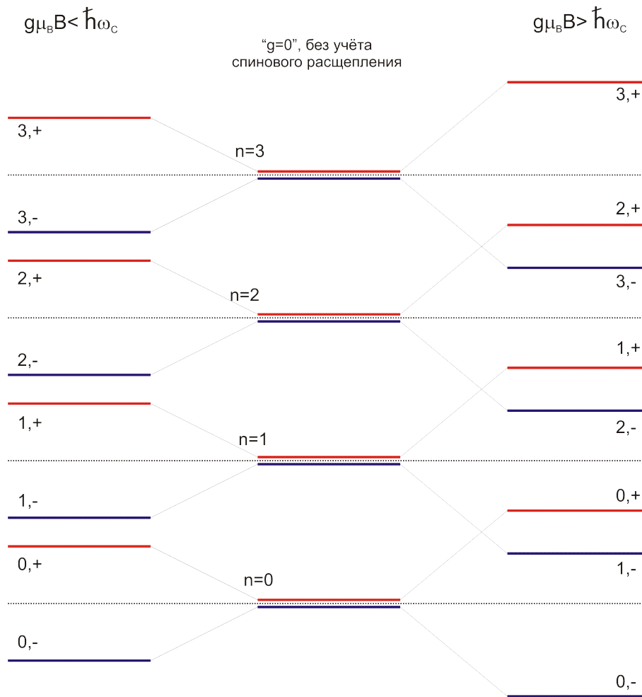
Рисунок 23: Схема чередования уровней Ландау с учётом спинового вырождения. В центре: без учёта зеемановского расщепления, каждый уровень Ландау двукратно вырожден по проекции спина. Слева: циклотронное расщепление больше зеемановского. Справа: зеемановское расщепление больше циклотронного.
