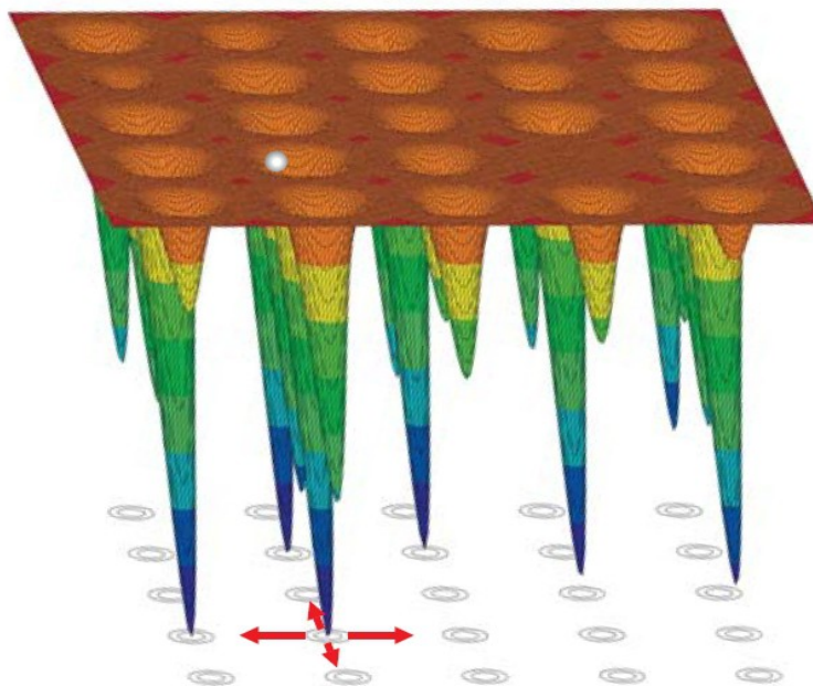
Рисунок 14 Схематическое представление случайной модуляции потенциала для электрона в кристалле. Из статьи [8].
