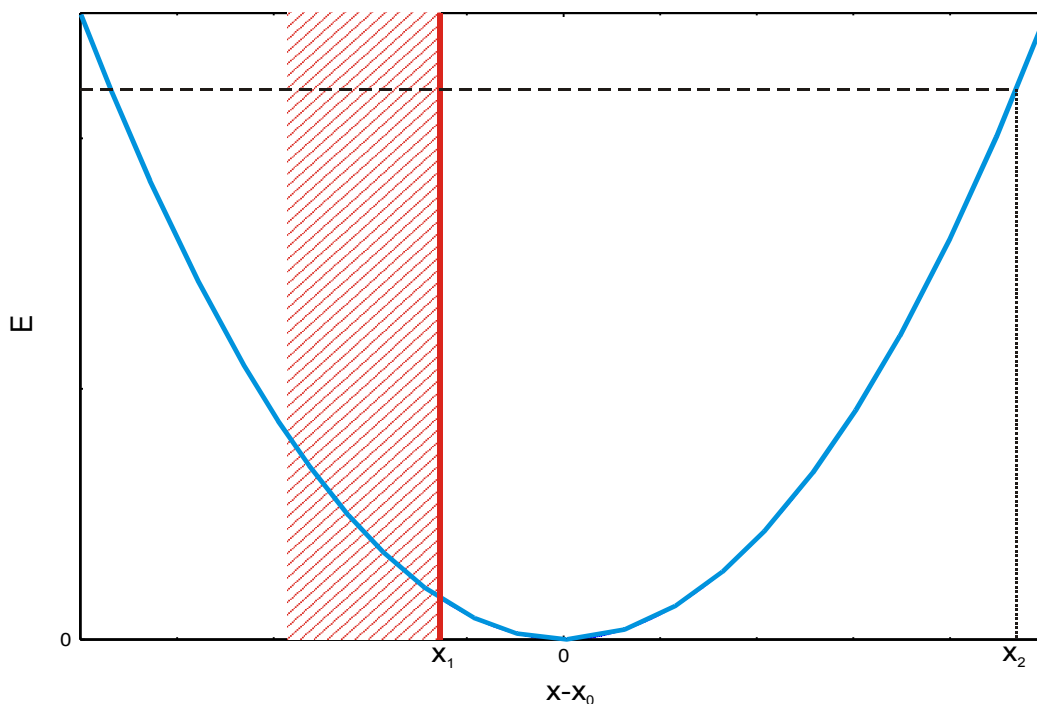
Рисунок 25: Потенциал гармонического осциллятора с запрещённой областью при x < x_1 .
