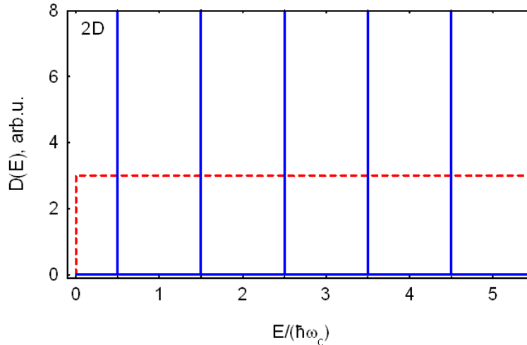
Рисунок 24: Плотность состояний как функция энергии (схематически) в трёхмерном (сверху) и двумерном (снизу) случае. Сплошная линия — с учётом квантования уровней Ландау, пунктир — в отсутствие магнитного поля. Спиновое расщепление не учитывается.
