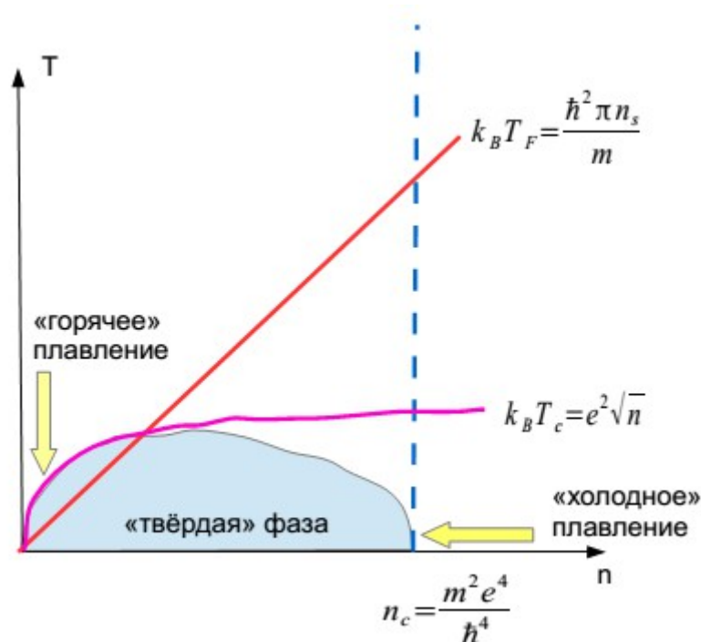
Рисунок 16: Схематическое построение фазовой диаграммы вигнеровского кристалла
