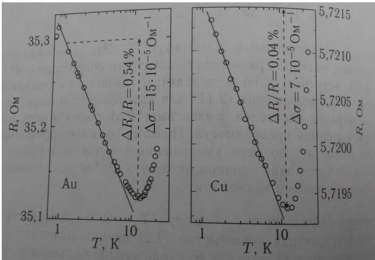
Рисунок 4: Температурные зависимости сопротивления тонких пленок меди и золота при низких температурах, демонстрирующие возникновение интерференционных поправок к проводимости. Из книги [2].
