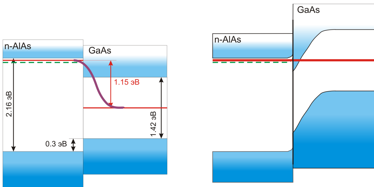
Рисунок 6: Построение энергетической диаграммы для гетероперехода между сильно легированным n-AlAs и чистым GaAs. Ширина запрещенной зоны и разрывы зон показаны в масштабе.
