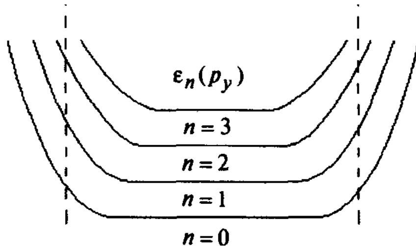
Рисунок 26: Схематическая зависимость положения уровня Ландау от координаты ведущего центра x_0 = \frac{\hbar c k_y}{eH} . Пунктиром показаны границы образца. Из книги [1].
