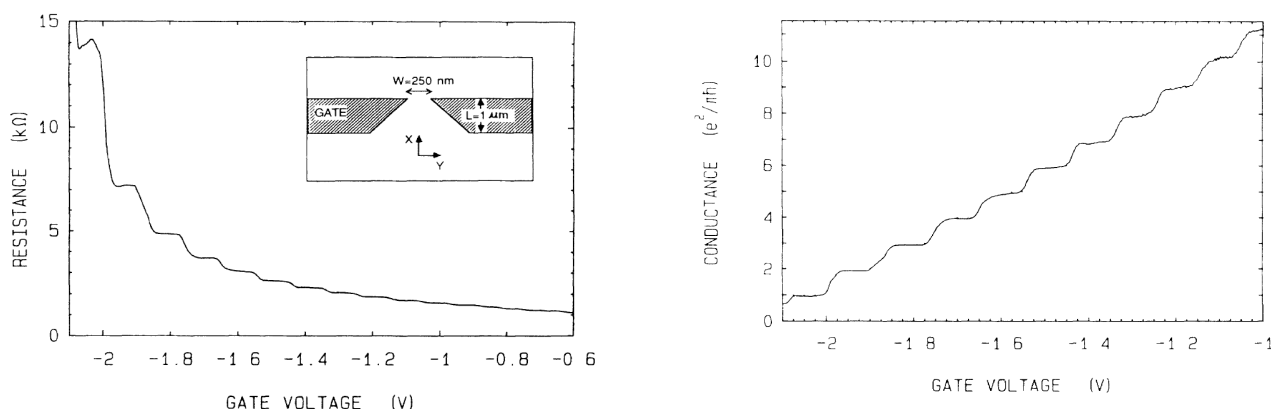
Рисунок 20: Слева: зависимость сопротивления точечного контакта от напряжения на затворе, на вставке показана схема точечного контакта. Справа: квантование проводимости (в единицах 2 \frac{e^2}{h} ) как функция напряжения на затворе. Температура опыта 0.6K. Из работы [22].
