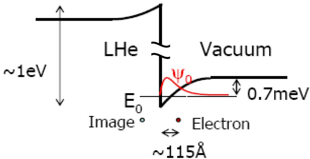
Рисунок 5: Схематическое изображение потенциала, действующего на электрон над поверхностью гелия. Из [14].
