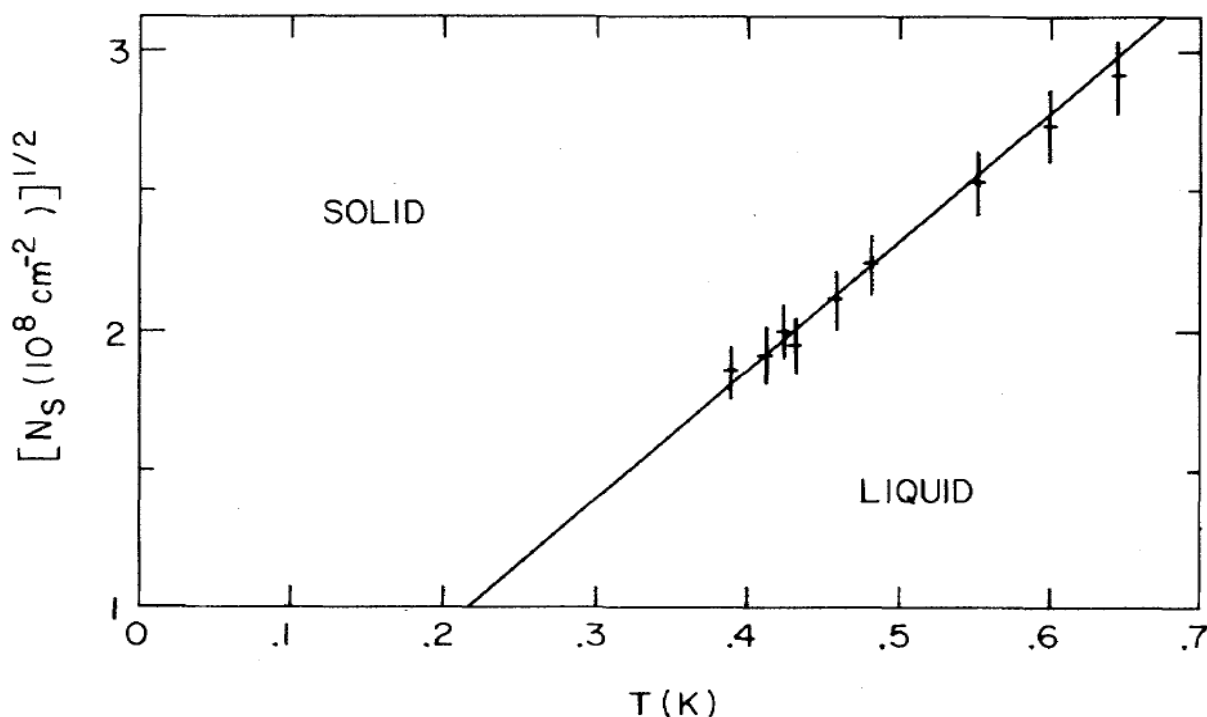
Рисунок 18: Фазовая диаграмма для двумерного электронного газа над поверхностью гелия. Из работы [21].
