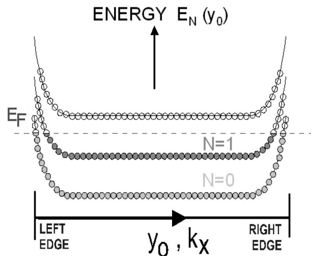
Рисунок 28: Схема заполнения уровней Ландау с учётом искривления уровней на границе образца. Из статьи [7]. Обозначения отличаются от обозначений нашего курса заменой y на x .
