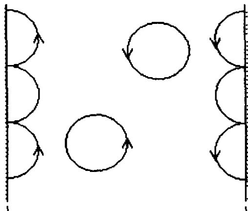
Рисунок 27: Замкнутые и скачущие циклотронные орбиты. Схематический рисунок. Из книги [1].
