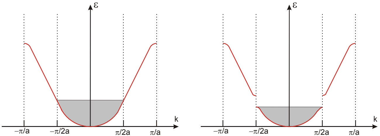
Рисунок 15: Схема заполнения электронных состояний до (слева) и после (справа) димеризации цепочек.
