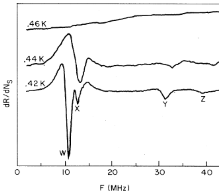
Рисунок 17: Экспериментальные записи линии, демонстрирующие возникновение плазмон-риплонных резонансов. Из работы [21]
